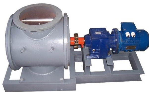
Шлюзовой затвор ШУ-15
